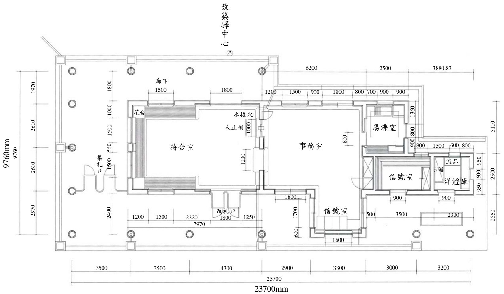
車站平面圖
