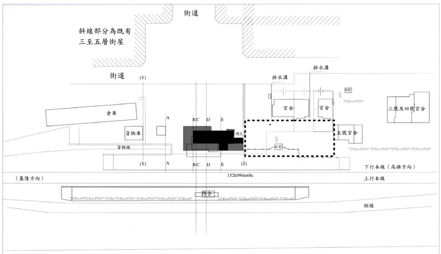
基地配置圖
